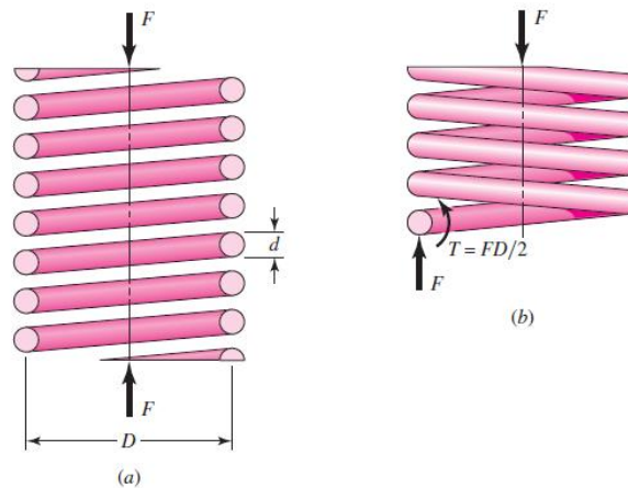
Figura 44 (a) Mola helicoidal carregada longitudinalmente (b) Diagrama de corpo livre indicando as duas componentes atuando no arame do fio (cisalhamento direto e torcional). Fonte: Shigley (2005)
