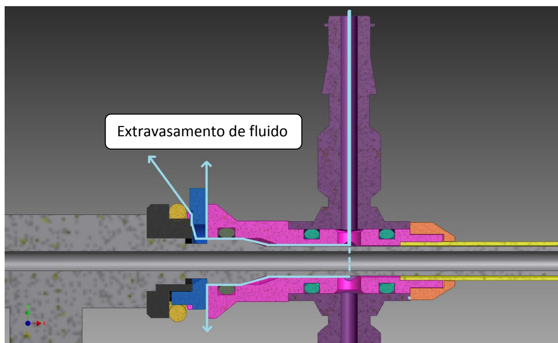
Figura 25 Indicação de possível extravasamento de fluido através do anel elástico interno
