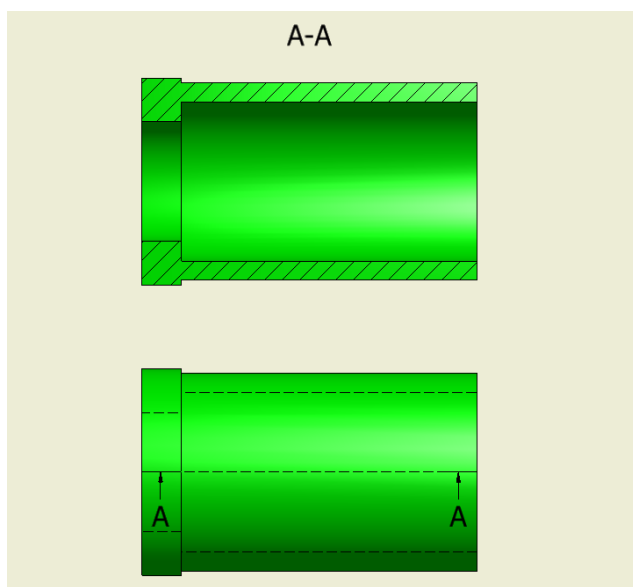
Figura 40 Vista em corte do empurrador
