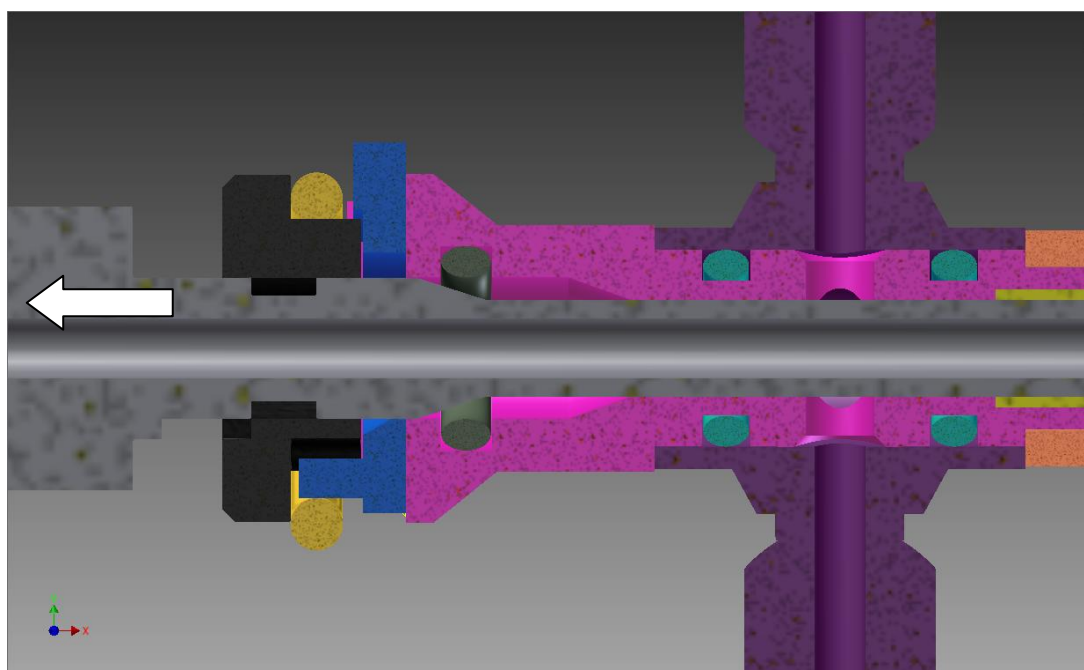
Figura 24 Recuo do artroscópio
