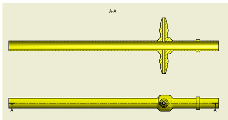
Figura 38 Vista em corte da cânula
