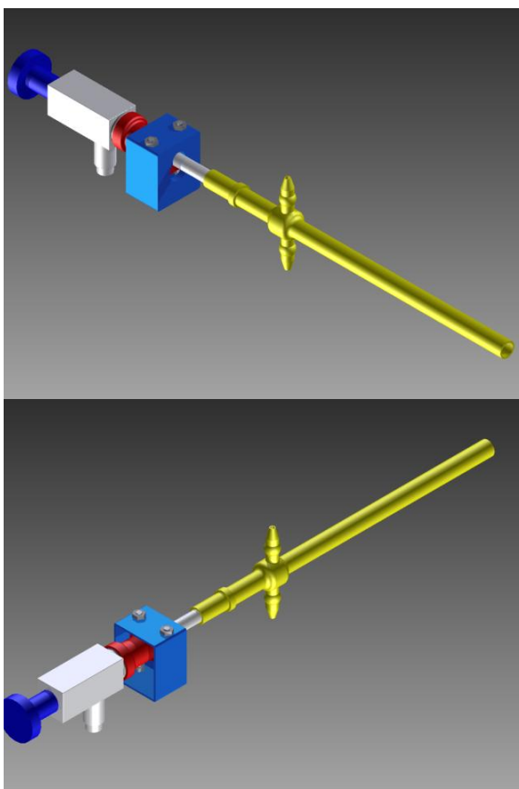
Figura 34 Sistema de acoplamento proposto
