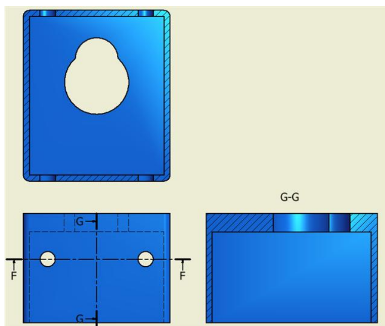
Figura 46 Vista em corte do deslizador
