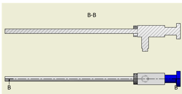
Figura 36 Vista em corte da óptica
