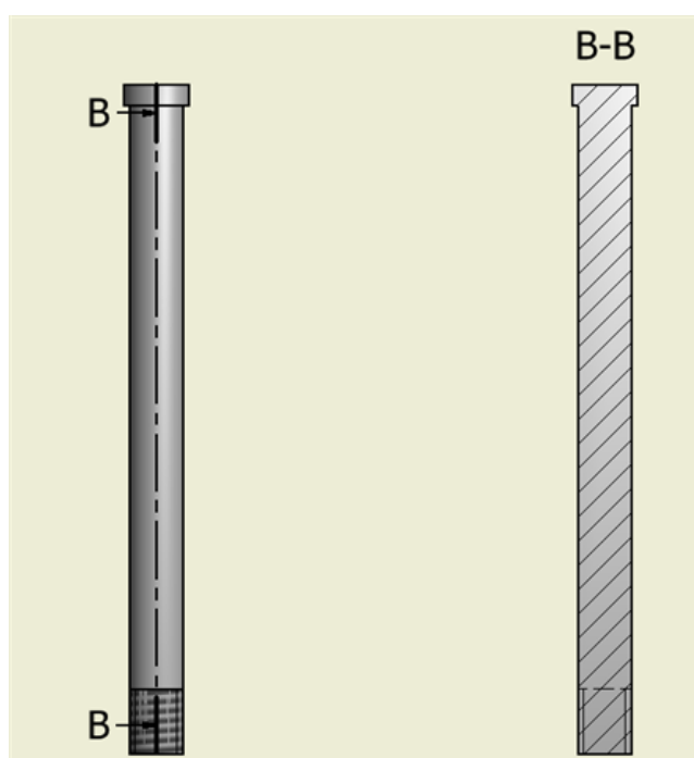
Figura 49 Vista em corte do pino
