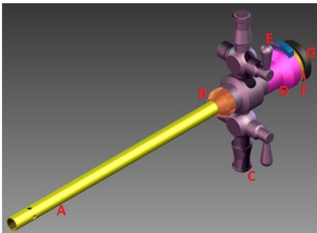
Figura 15 Modelo da cânula Stryker
