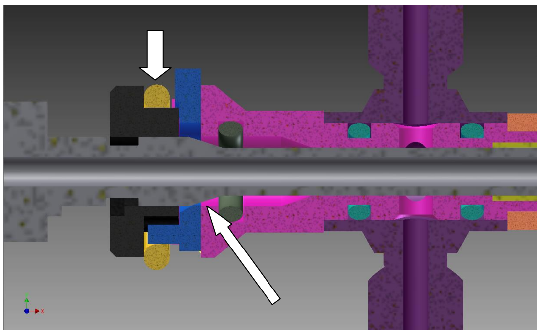
Figura 20 A região cônica do artroscópio desloca o elemento deslocador para baixo (contra a força do anel elástico)
