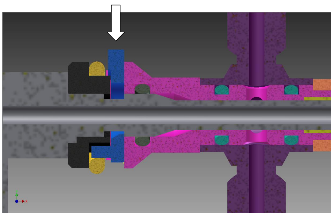
Figura 23 Acionamento manual do elemento deslocador para o destravamento
