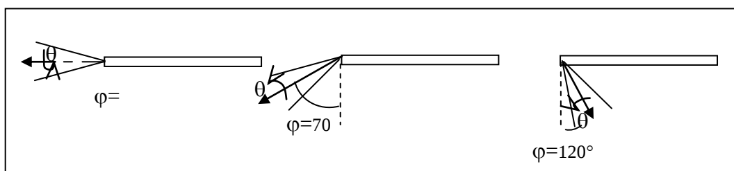
Figura 2 Graus de liberdade de um artroscópio rígido
