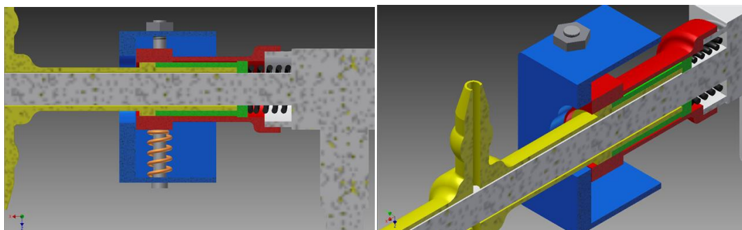
Figura 55 Início do deslocamento do deslizador
